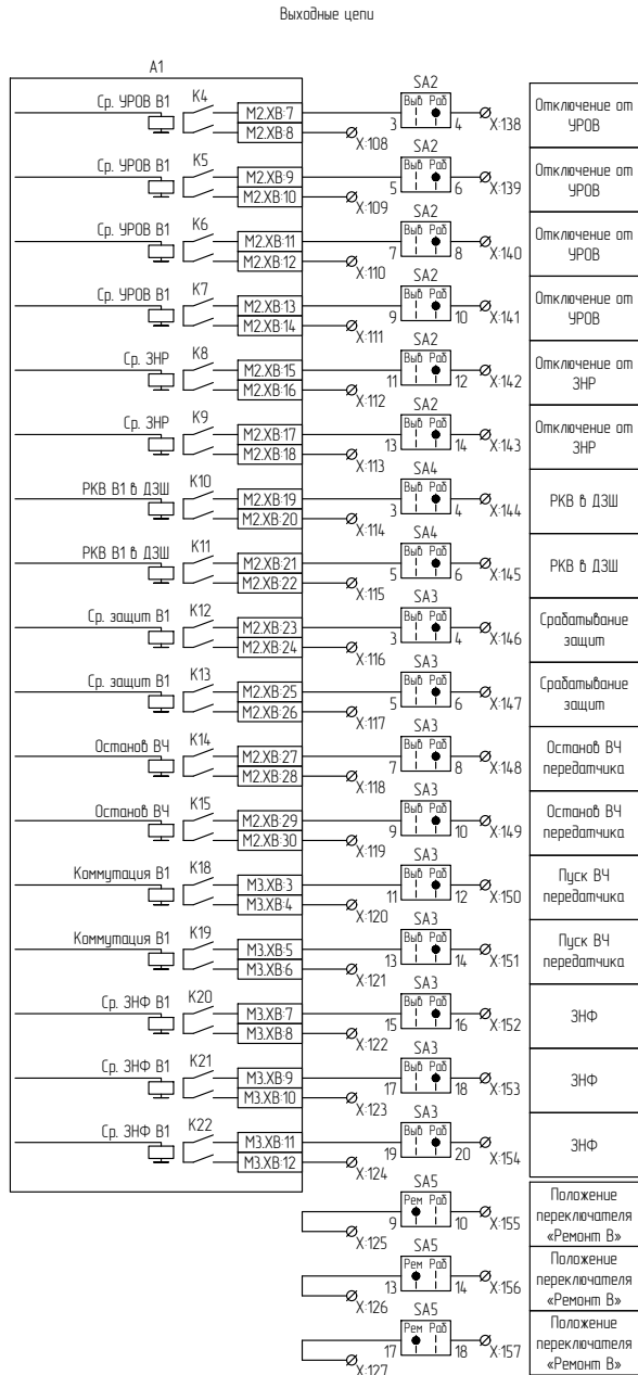
Рисунок В.4 – Схема электрическая принципиальная (часть 4)
