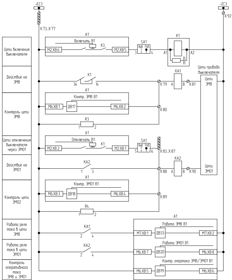
Рисунок В.3 – Схема электрическая принципиальная (часть 3)
