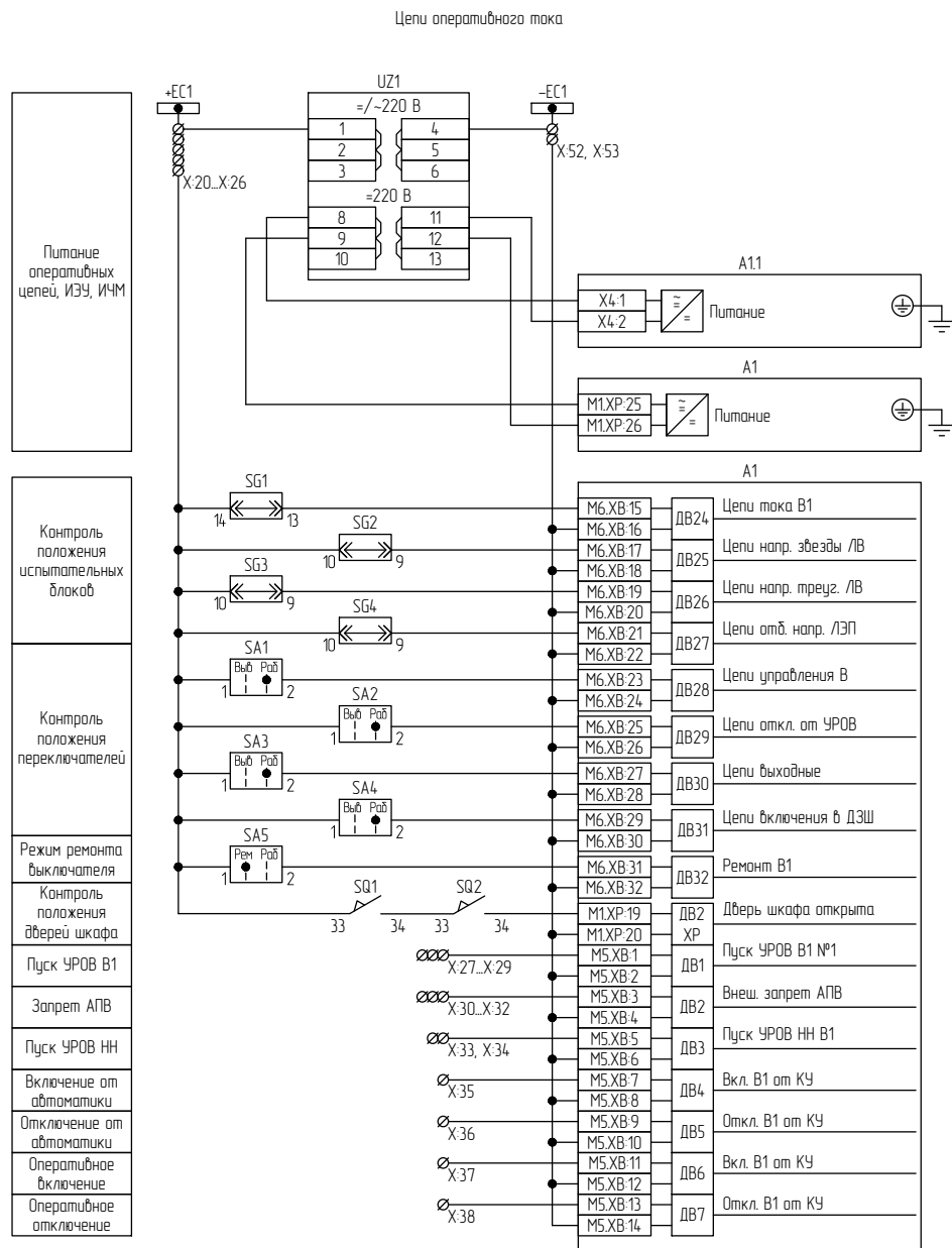
Рисунок В.2 – Схема электрическая принципиальная (часть 2)
